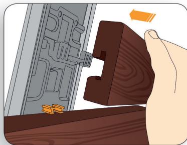
5 : Pose de la lame suivante
