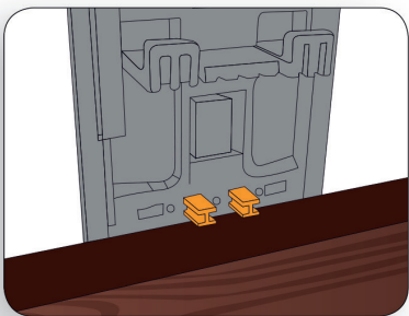
4 : Serrage de la lame à l'insertion du deuxième clip
